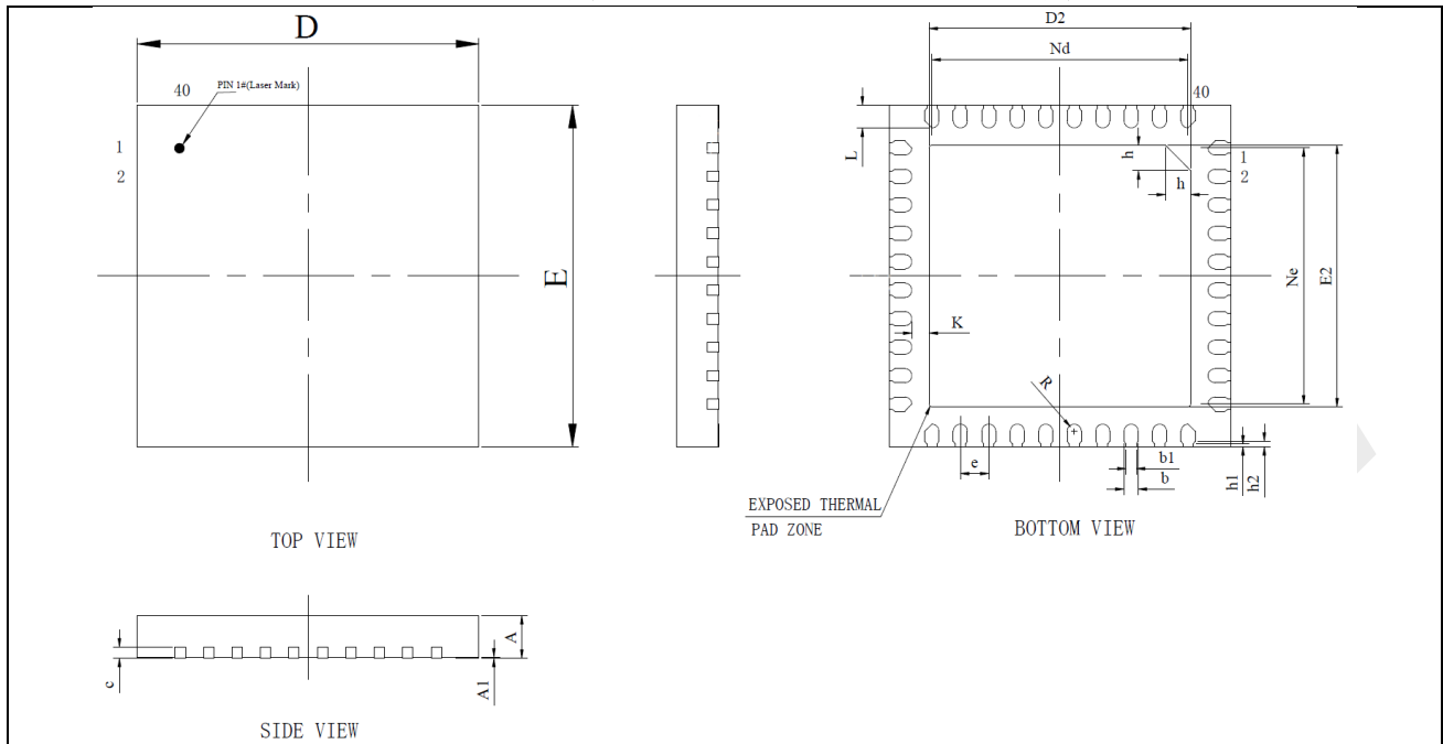
图 7-3: QFN40 – 40 脚, 6mm x 6mm 方形扁平无引脚封装图
