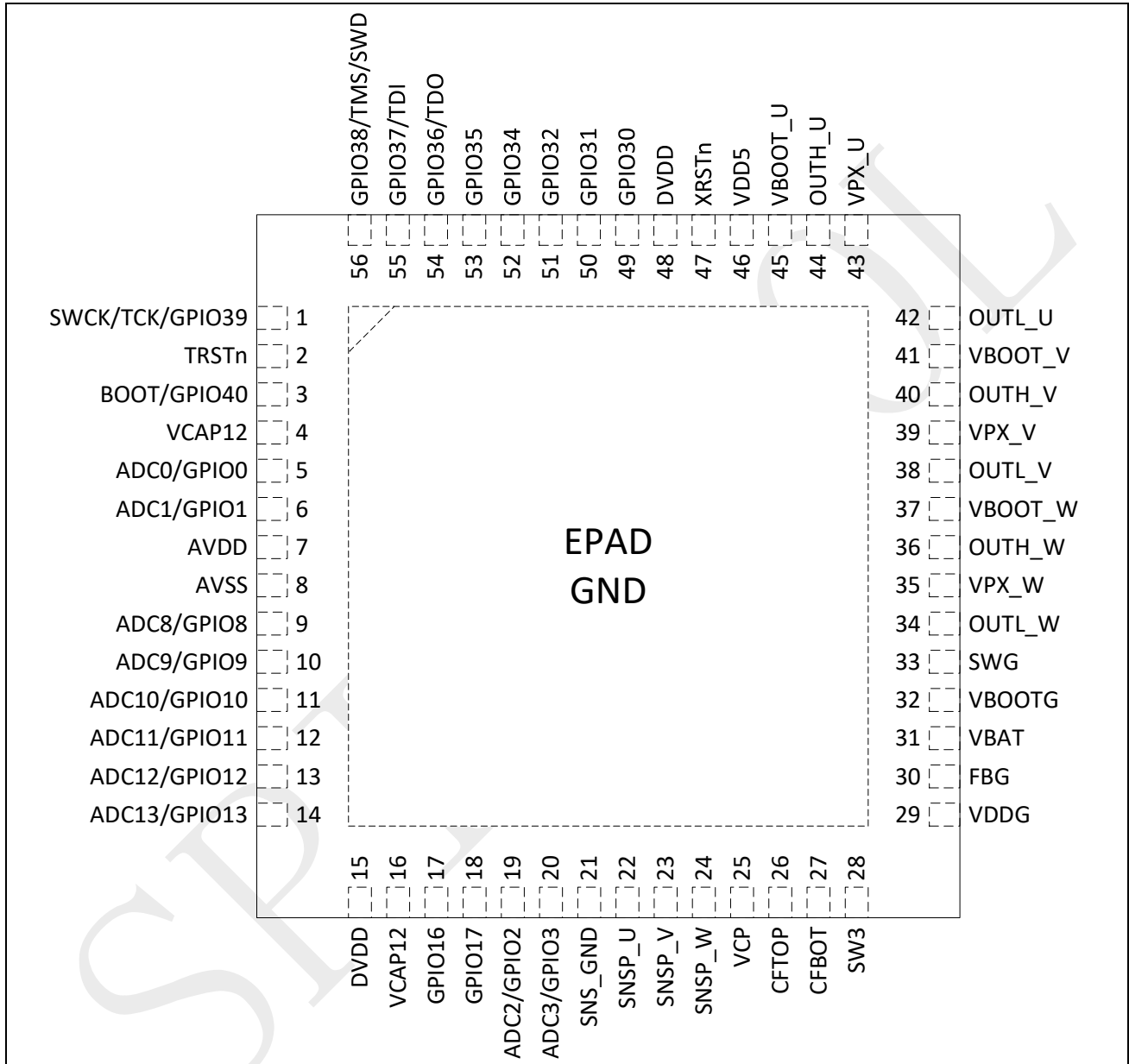
图 3-1: SPD1188 QFN56 引脚排列
