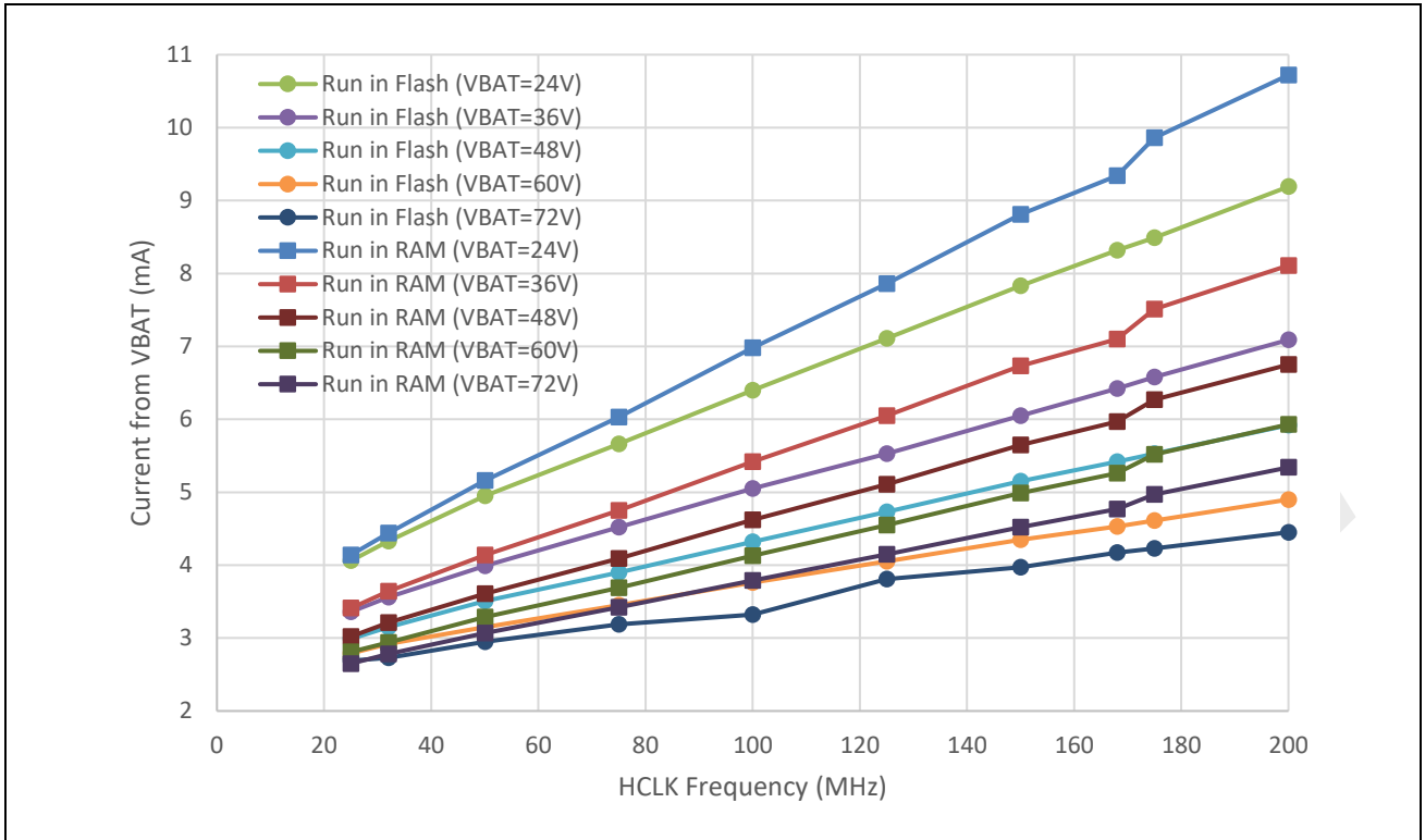
图 5-1: 典型工作电流随频率变化关系
