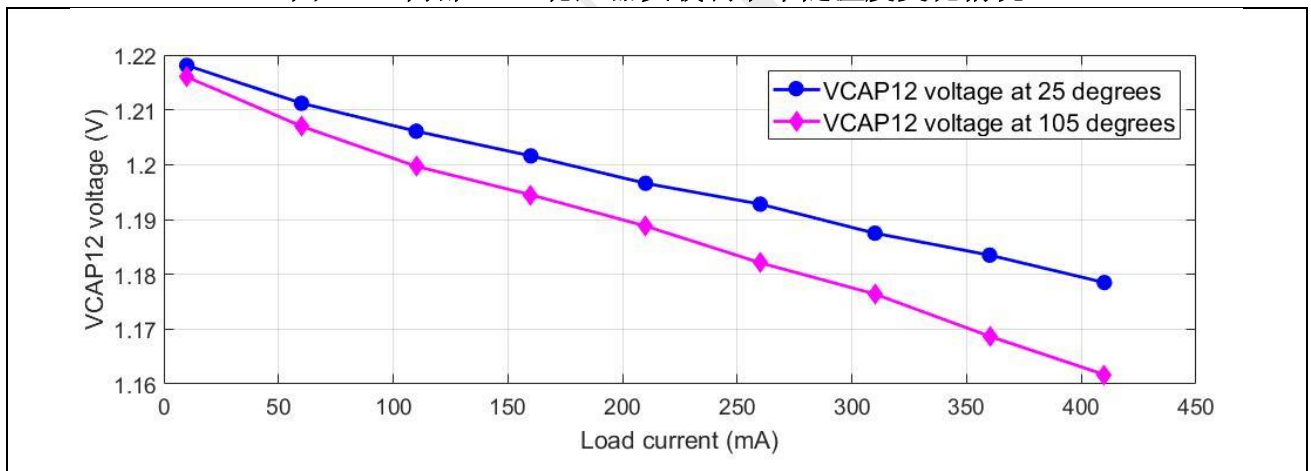
图 5-3: 内部 1.2V 稳压器负载调节率随温度变化情况
