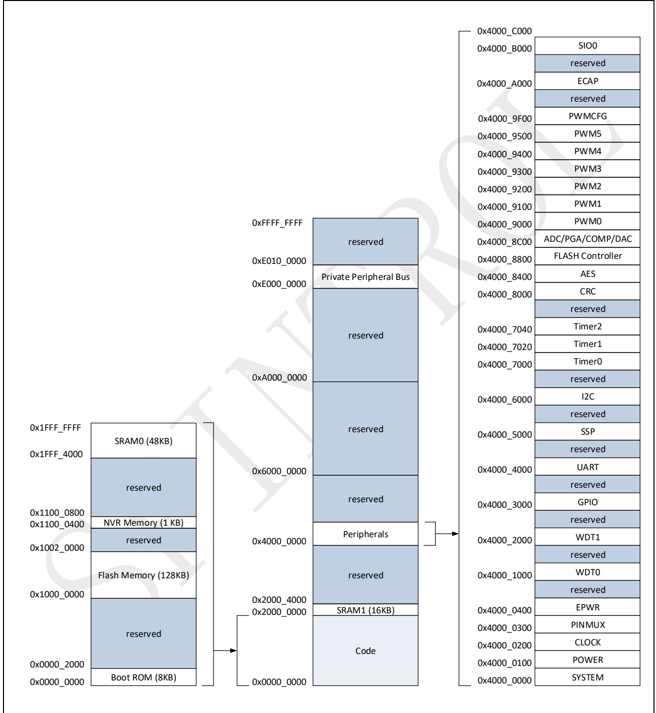
图 4-1: 存储器映射
