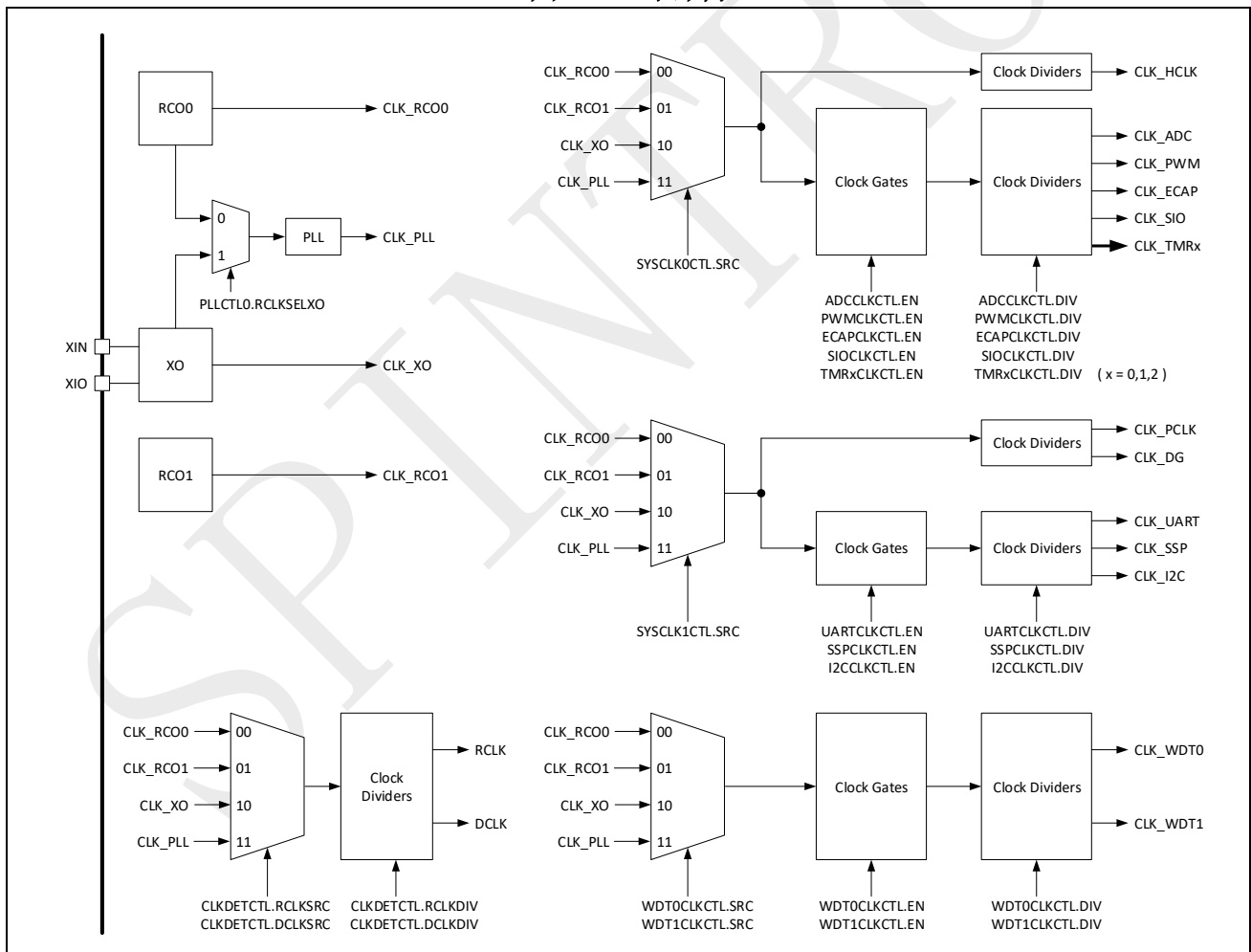
图 1-2: 时钟树
