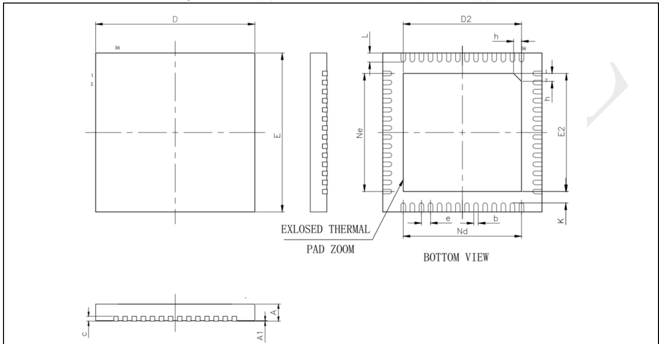
图 7-1: QFN56 – 56 脚, 7mm x 7mm 方形扁平无引脚封装图
