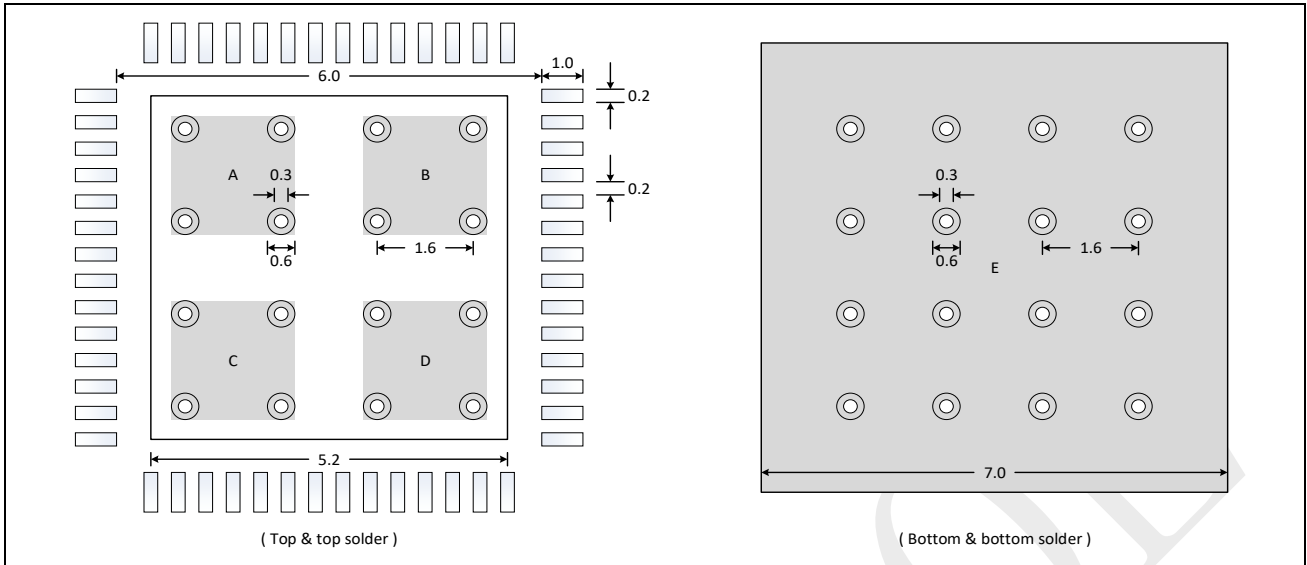
图 7-2: QFN56 – 56 脚, 7mm x 7mm 方形扁平无引脚封装建议尺寸
