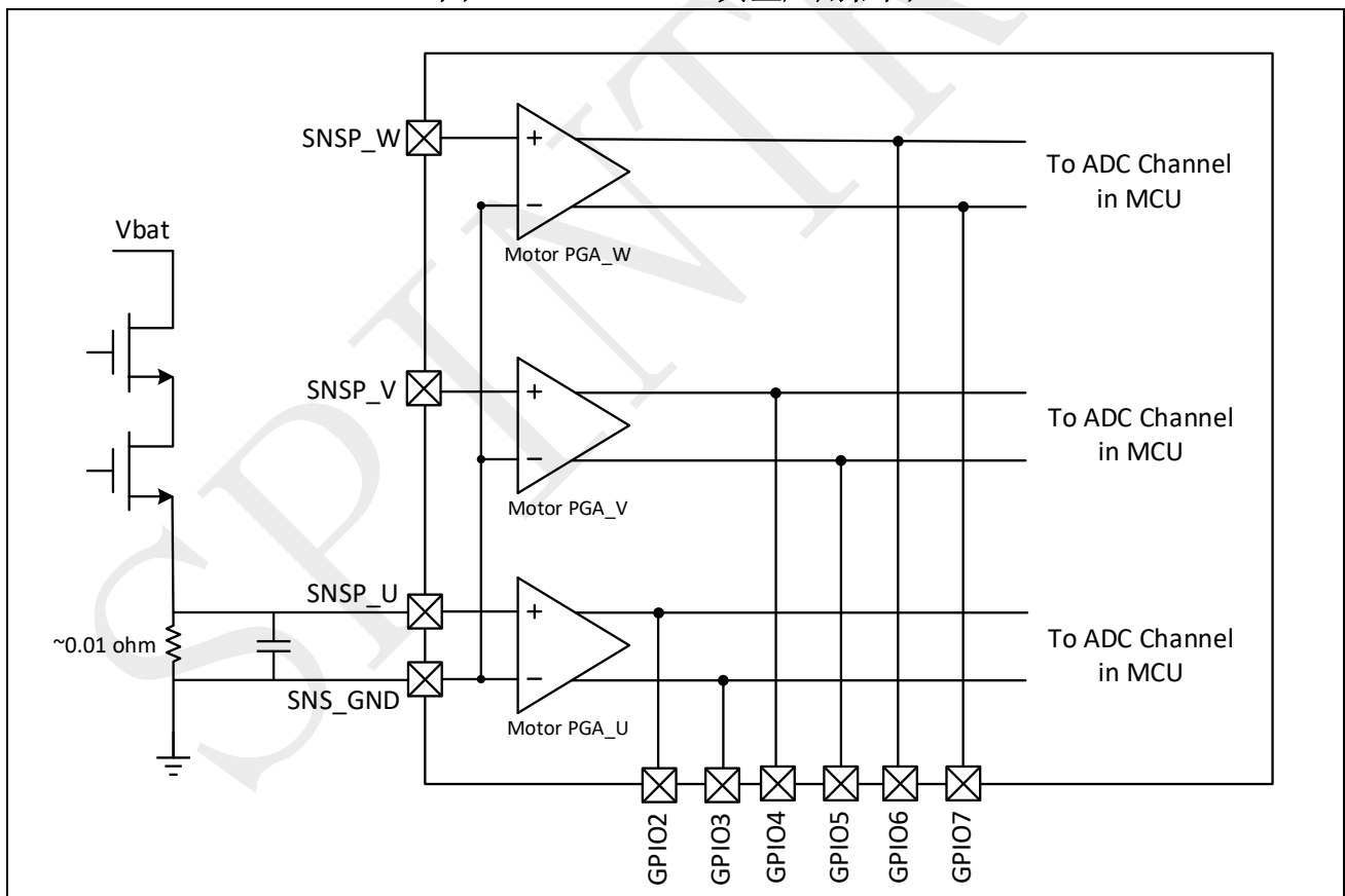
图 2-1: Motor PGA 典型应用框图
