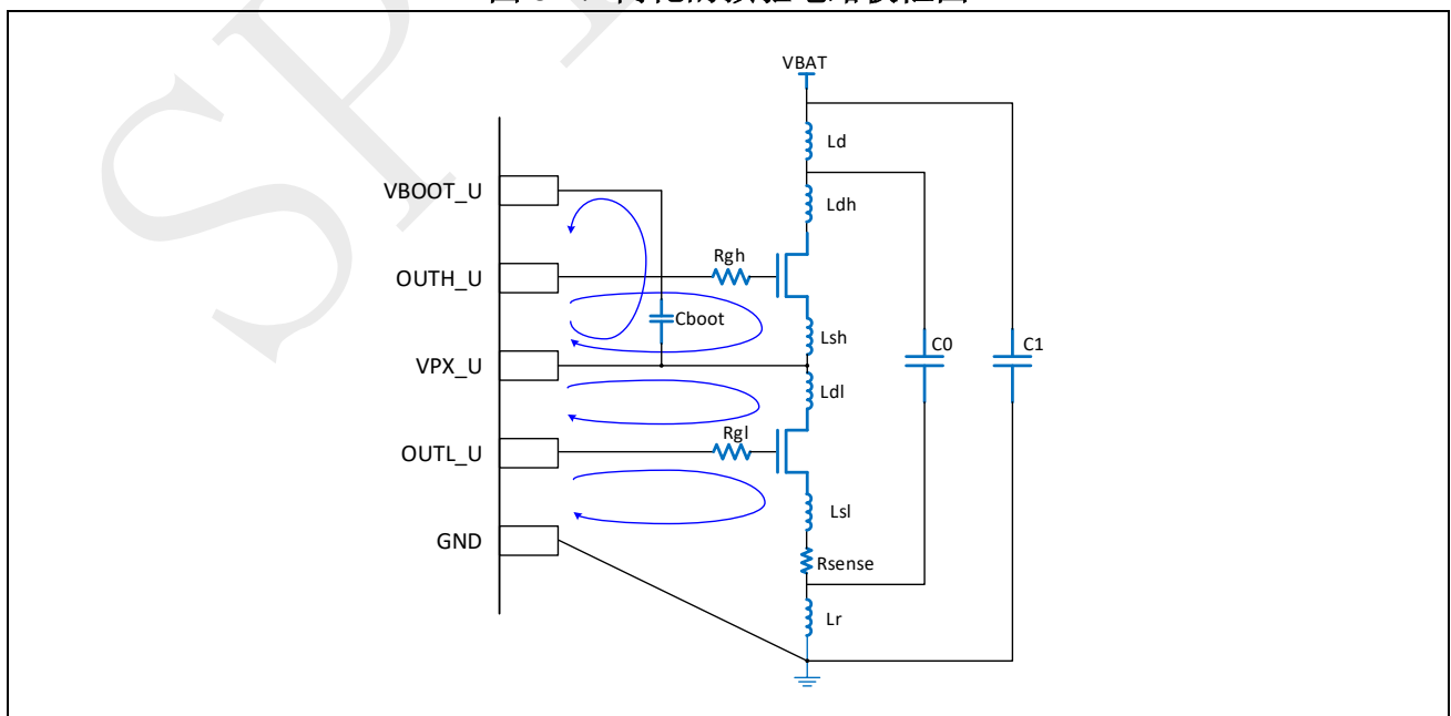
图 6-1: 简化的预驱电路板框图
