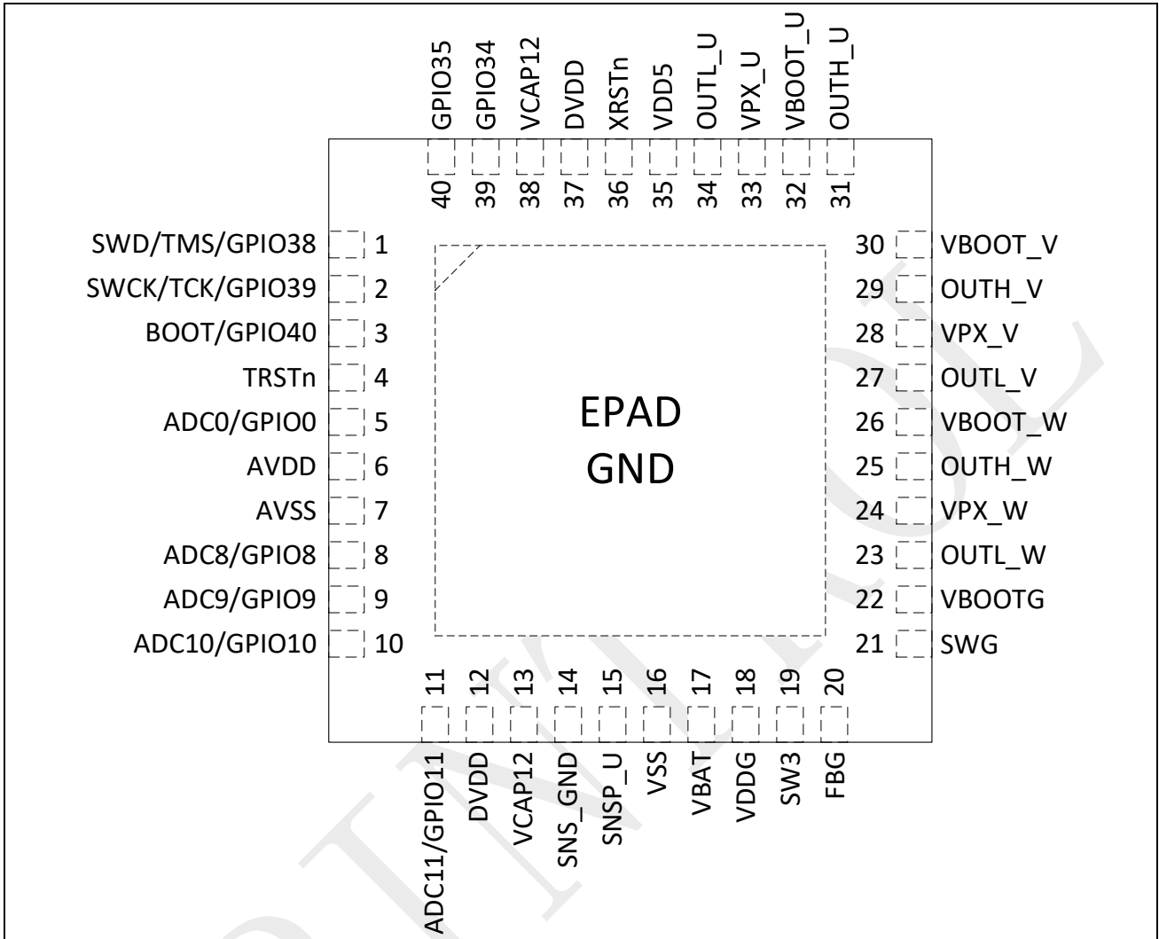
图 3-2: SPD1188 QFN40 引脚排列
