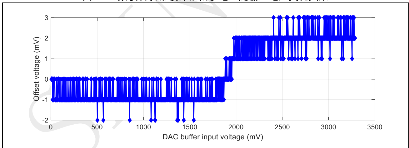
图 5-8: 数模转换器缓冲器偏移电压随输入电压变化关系
