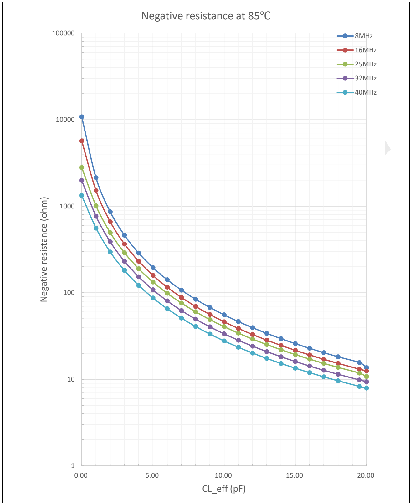
图 5-5: 内部晶振负阻值 (85 °C)
