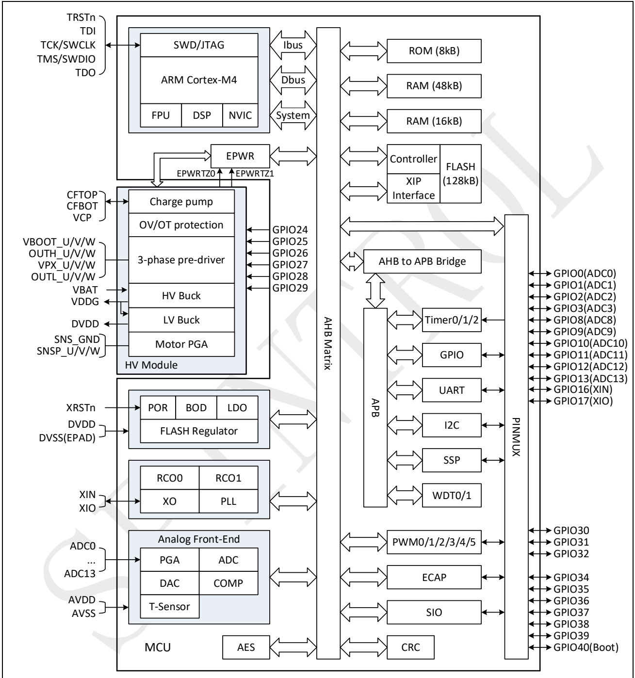
图 1-1: SPD1188 功能框图
